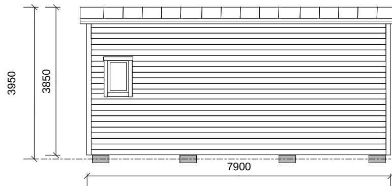
FASAD BAKSIDA
