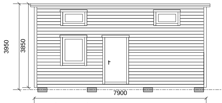
FASAD FRAMSIDA
